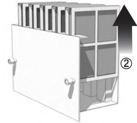
② 카트리지 내 필터 분리 Remove the filters from the cartilage
