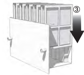
③ 교체 후 다시 장착 Exchange the filters and replace it in the cartilage
